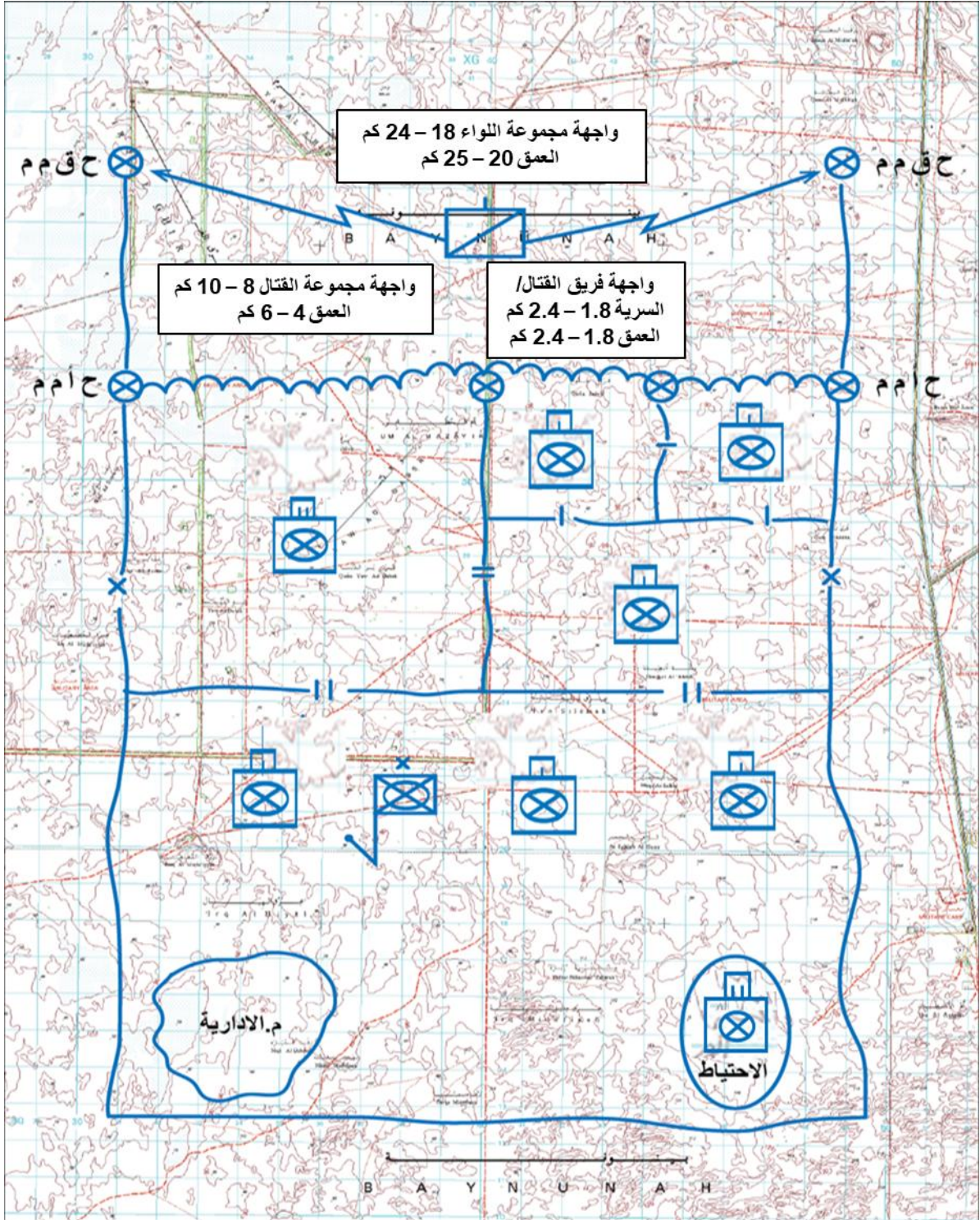
الشكل رقم (1) اتساع وعمق منطقة عمليات مجموعة القتال / الكتيبة
