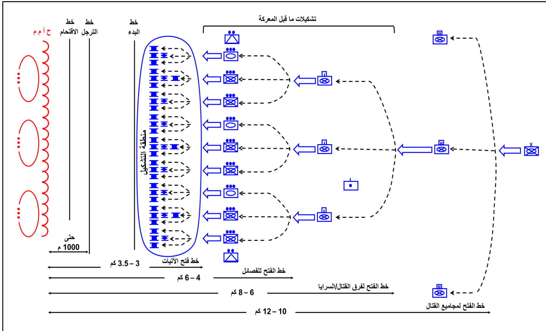
الشكل رقم (15) مثال على خطوط الفتح التعبوي
