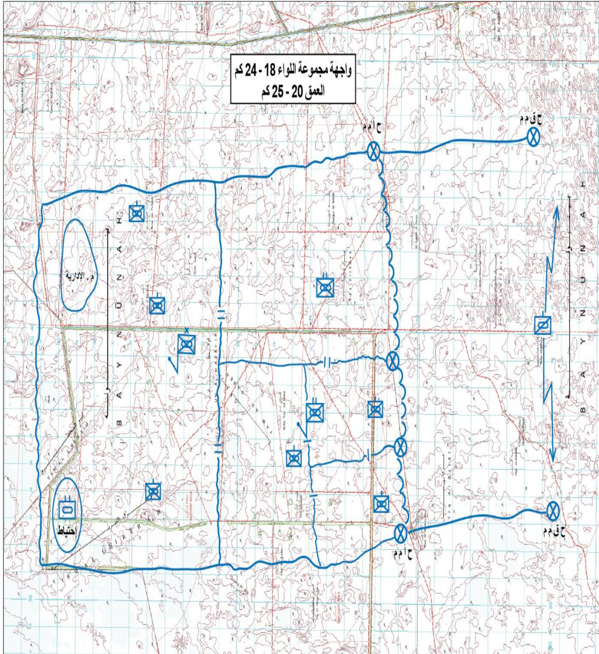
الشكل رقم (6) إجراءات السيطرة الدفاعية التخطيطية لمجموعة القتال/ الكتيبة ضمن مجموعة اللواء
