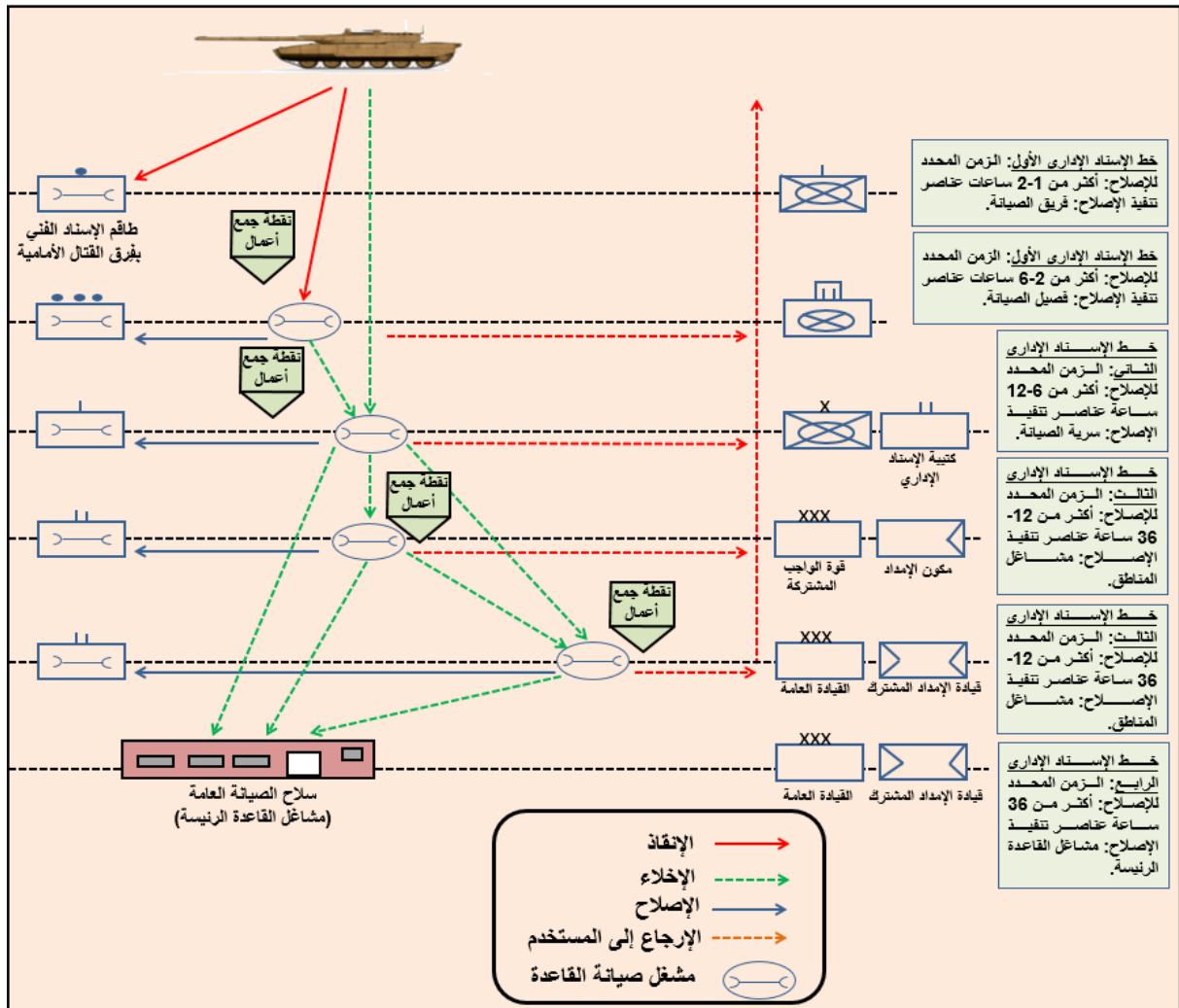
الشكل رقم (43) مخطط الإنقاذ والإصلاح والإخلاء
